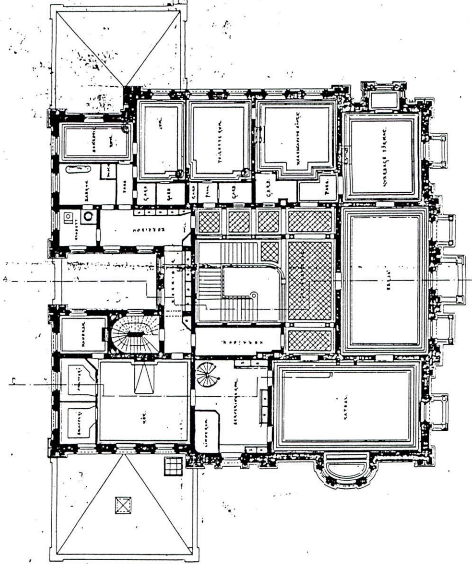
PLAN AF DEN VÄNDRINGEN.
